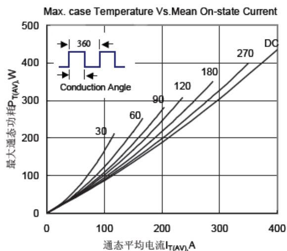
Fig.5 最大功耗与通态电流关系曲线
