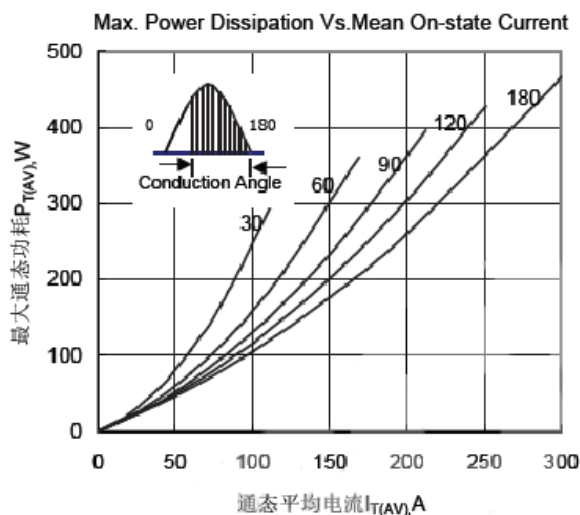
Fig.3 最大功耗与通态平均电流关系曲线
