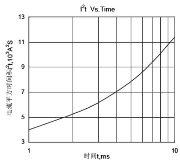
Fig.6 I^2t 特性曲线
